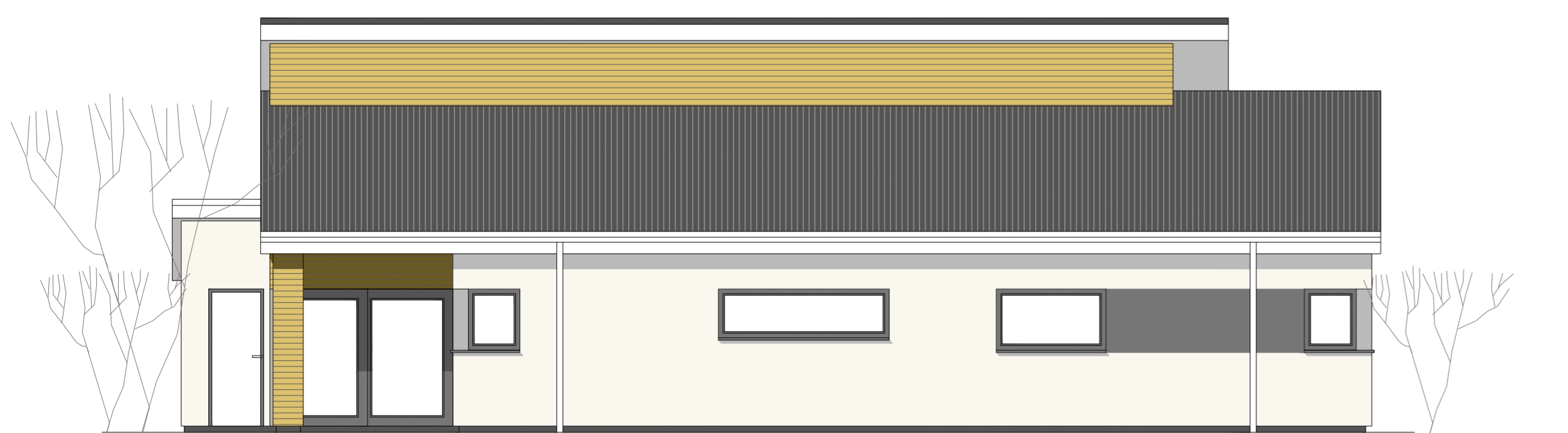
POHĽAD BOČNÝ M 1:75
